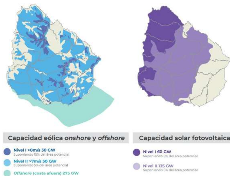
Figura 4 . Capacidades potenciales (GW) según fuente renovable.
