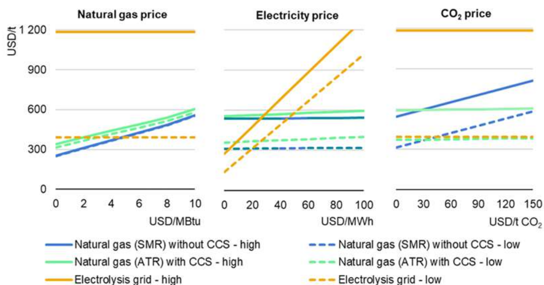
Figura 15. Costo nivelado de producción de amoníaco (LCOA) en diferentes vías de precios de gas, electricidad y CO 2
