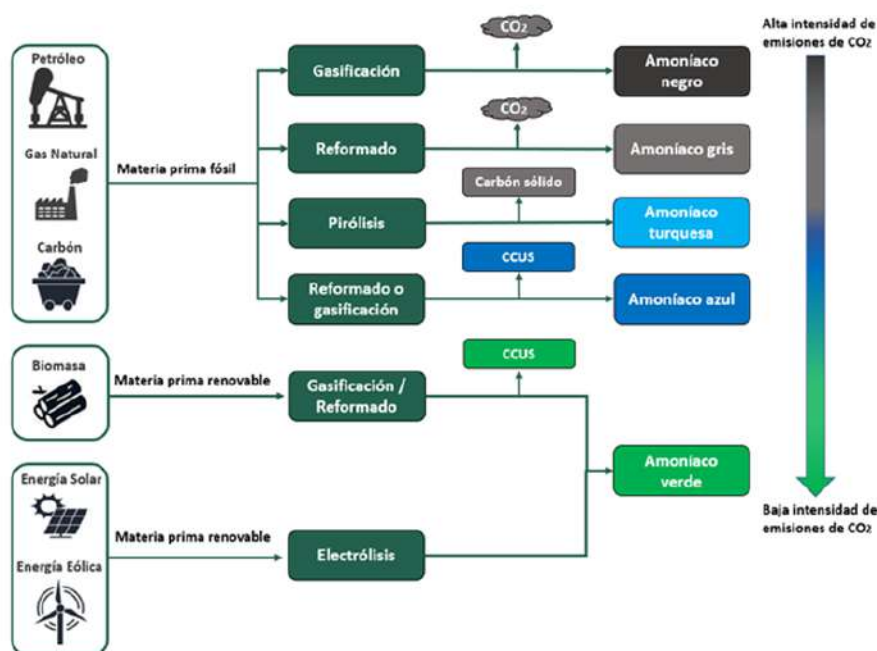
Figura 11. Tipo de amoníaco según su método de producción
