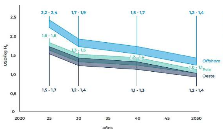
Figura 6 . Curva de costos nivelados de producción de hidrógeno en Uruguay (LCOH).
