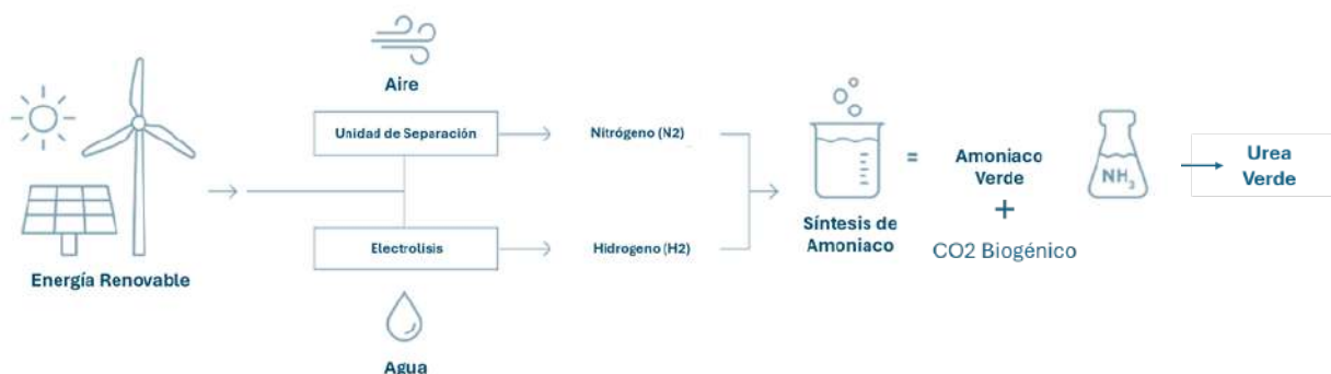
Figura 8. Tren de proceso de producción de amoníaco verde y urea Verde
