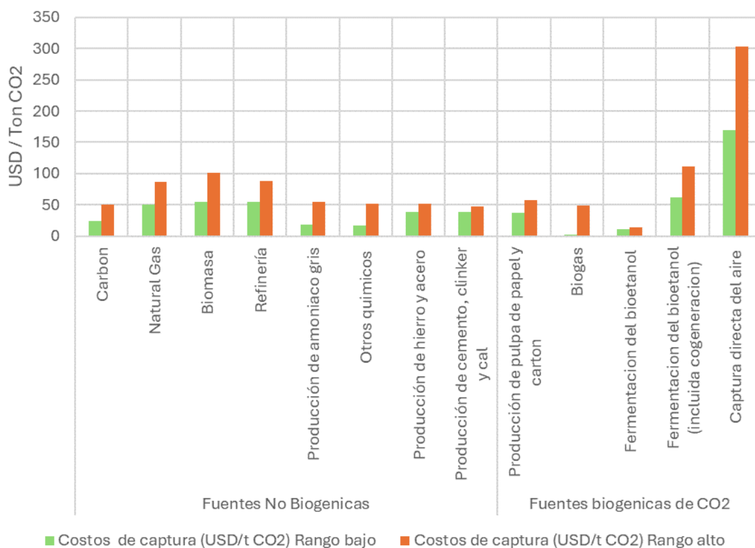
Figura 16. Costos de captura de CO 2 dependiendo de la fuente
